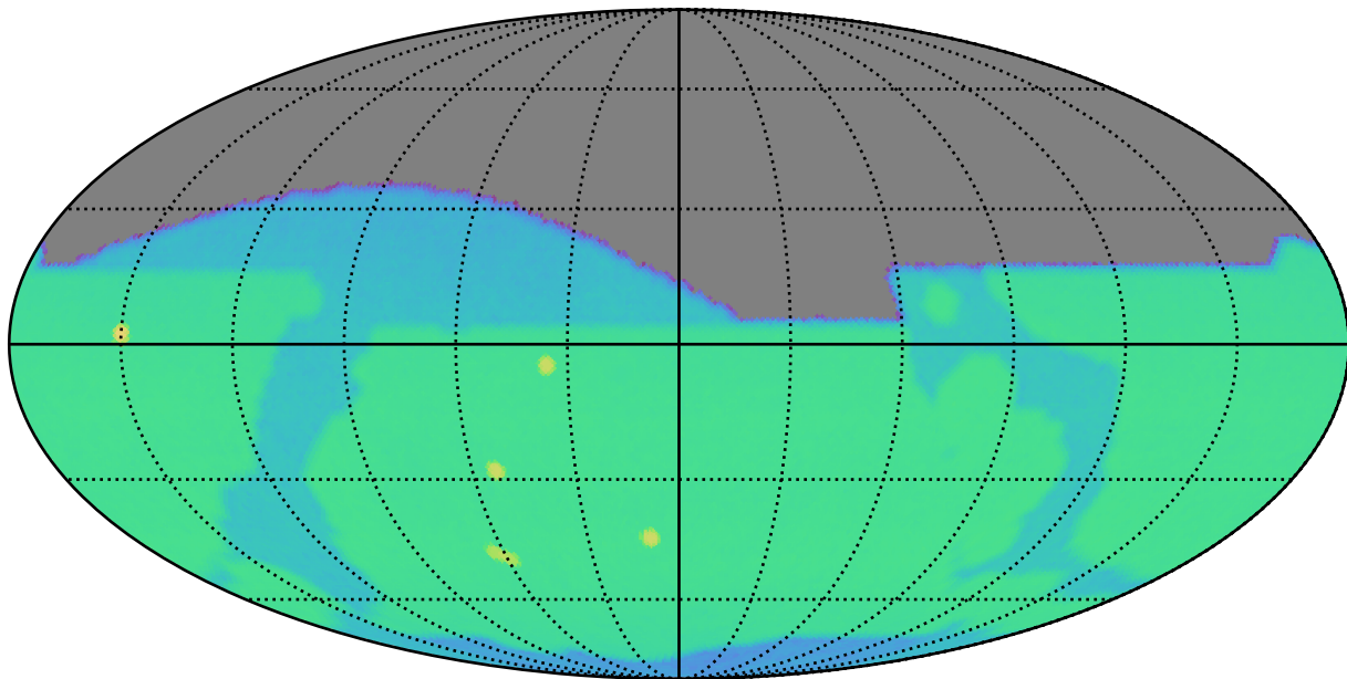
weather_cloudso8v3.4_10yrs i: SurfaceBrightLimit
