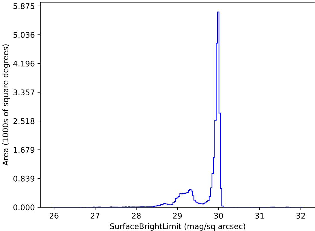
weather_cloudso8v3.4_10yrs i: SurfaceBrightLimit
