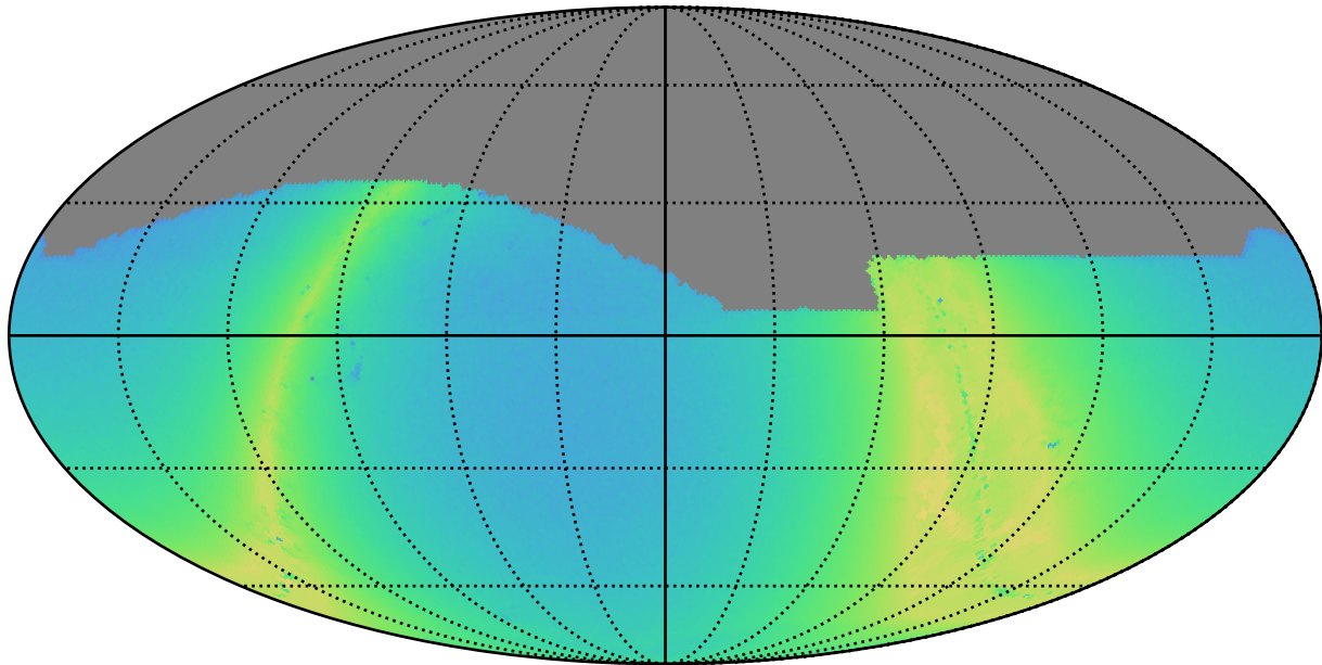
weather_cloudso8v3.4_10yrs i: N stars to Precision 0.20
