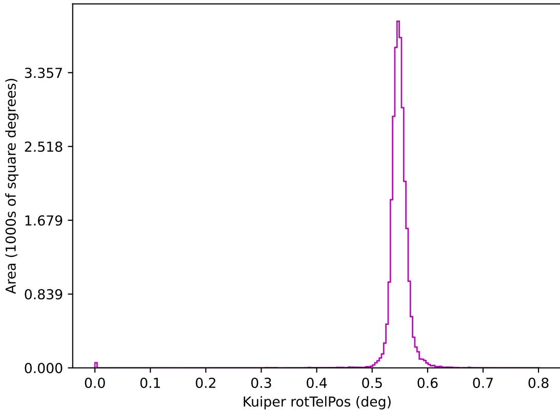
weather_cloudso8v3.4_10yrs z: Kuiper rotTelPos
