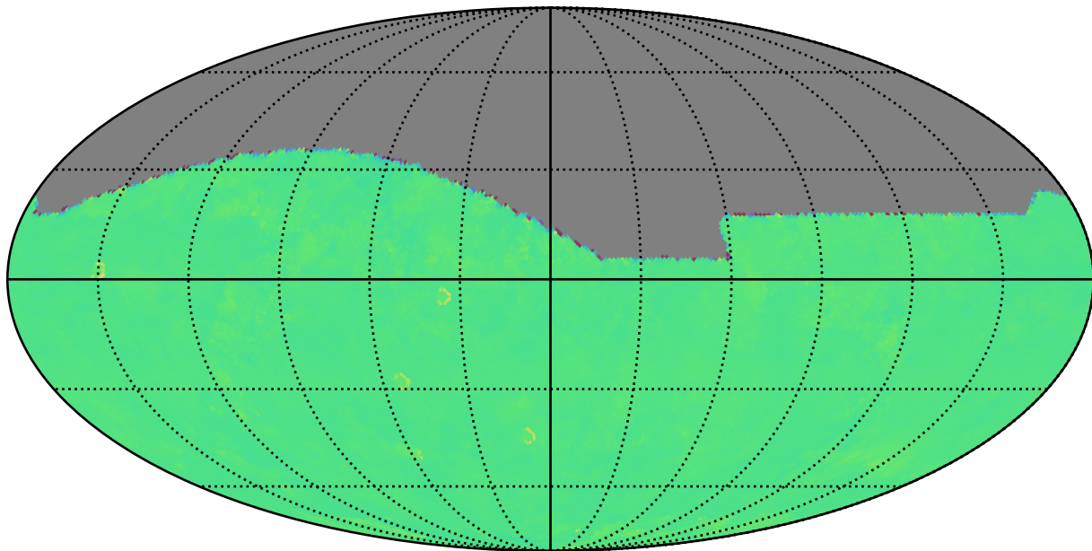
weather_cloudso8v3.4_10yrs r: Kuiper rotTelPos
