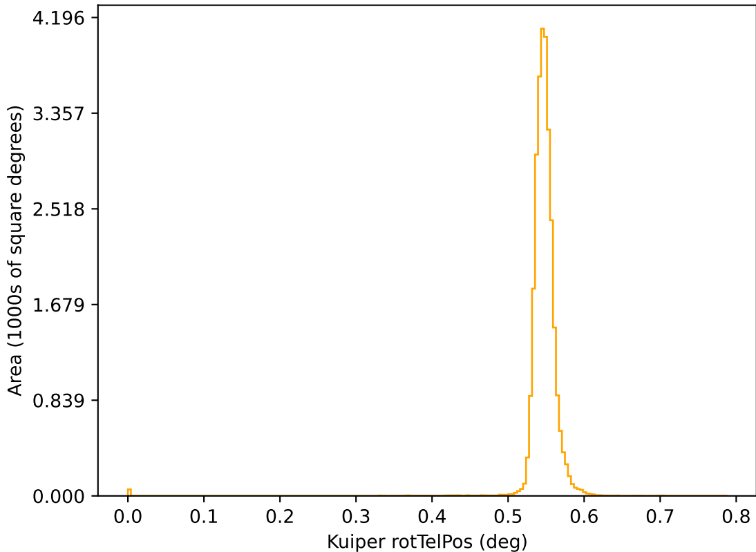
weather_cloudso8v3.4_10yrs r: Kuiper rotTelPos
