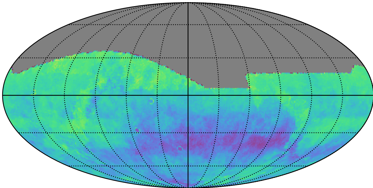
weather_cloudso8v3.4_10yrs z: Kuiper rotSkyPos
