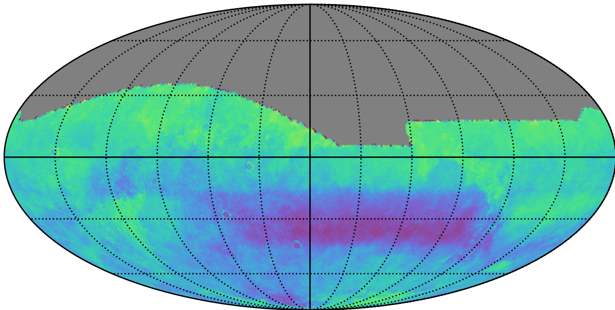
weather_cloudso8v3.4_10yrs r: Kuiper rotSkyPos
