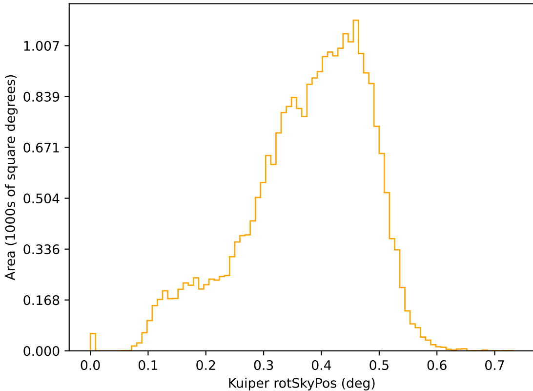
weather_cloudso8v3.4_10yrs r: Kuiper rotSkyPos
