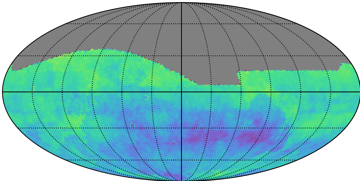
weather_cloudso8v3.4_10yrs i: Kuiper rotSkyPos
