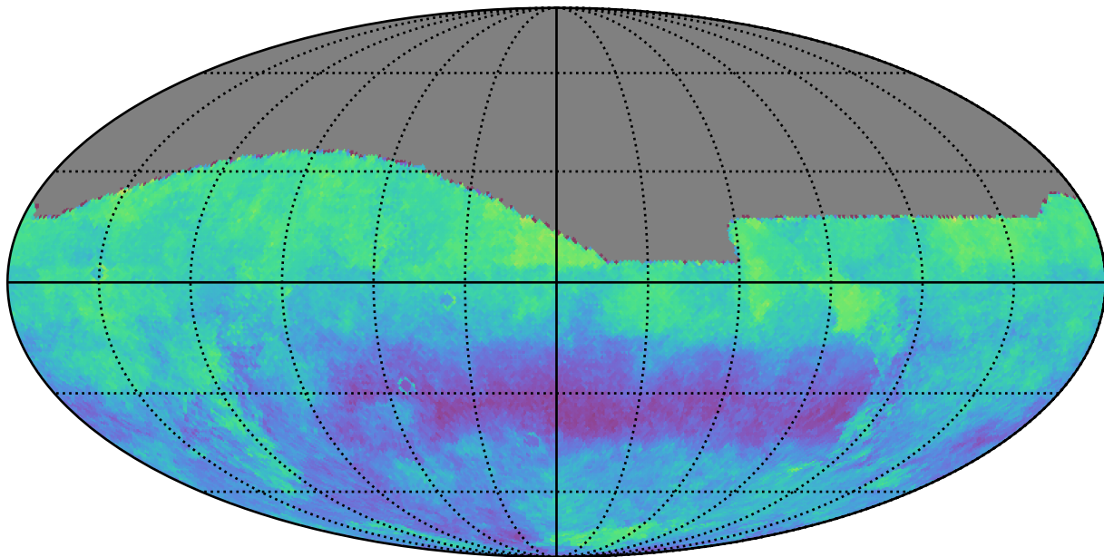
weather_cloudso8v3.4_10yrs g: Kuiper rotSkyPos
