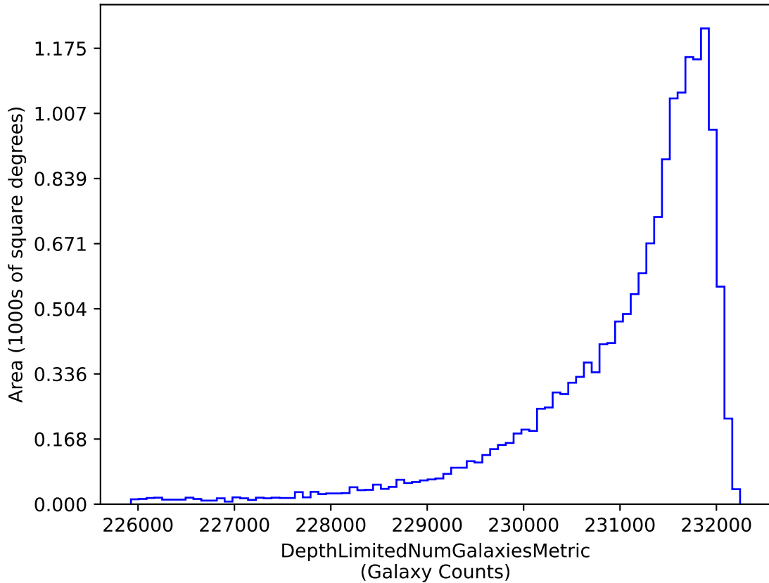
weather_cloudso8v3.4_10yrs i band galaxies non-DD: DepthLimitedNumGalaxiesMetric
