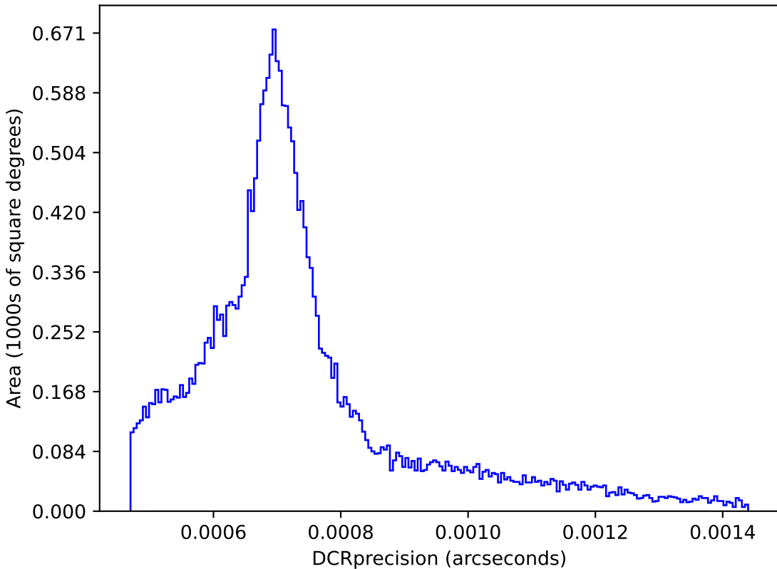
weather_cloudso8v3.4_10yrs : DCRprecision
