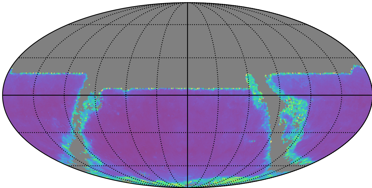
weather_cloudso8v3.4_10yrs y band: AGN SF_uncert
