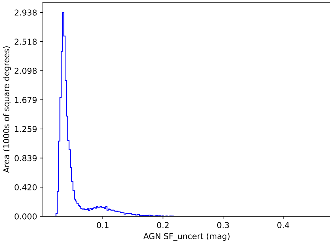
weather_cloudso8v3.4_10yrs y band: AGN SF_uncert
