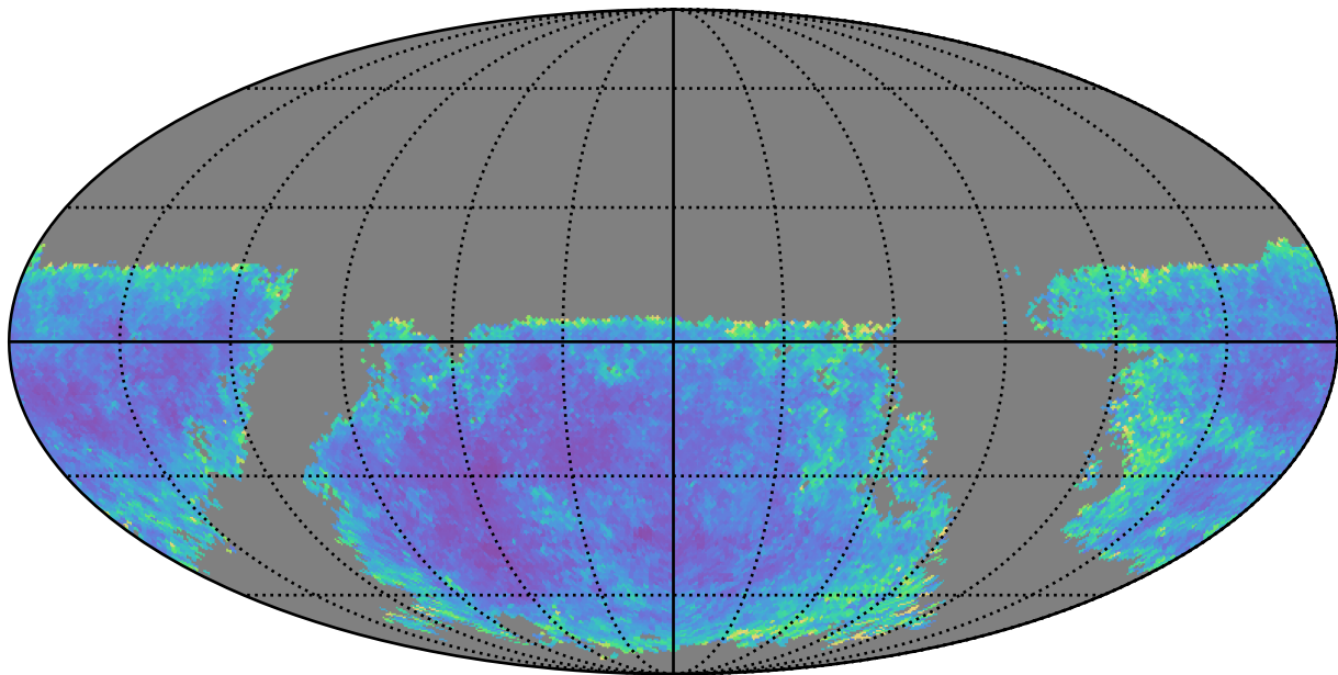
weather_cloudso8v3.4_10yrs u band: AGN SF_uncert
