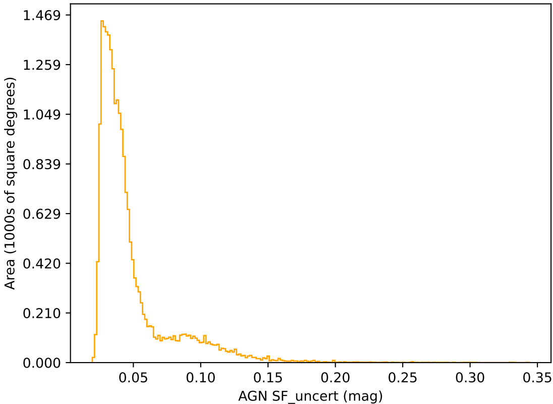
weather_cloudso8v3.4_10yrs r band: AGN SF_uncert
