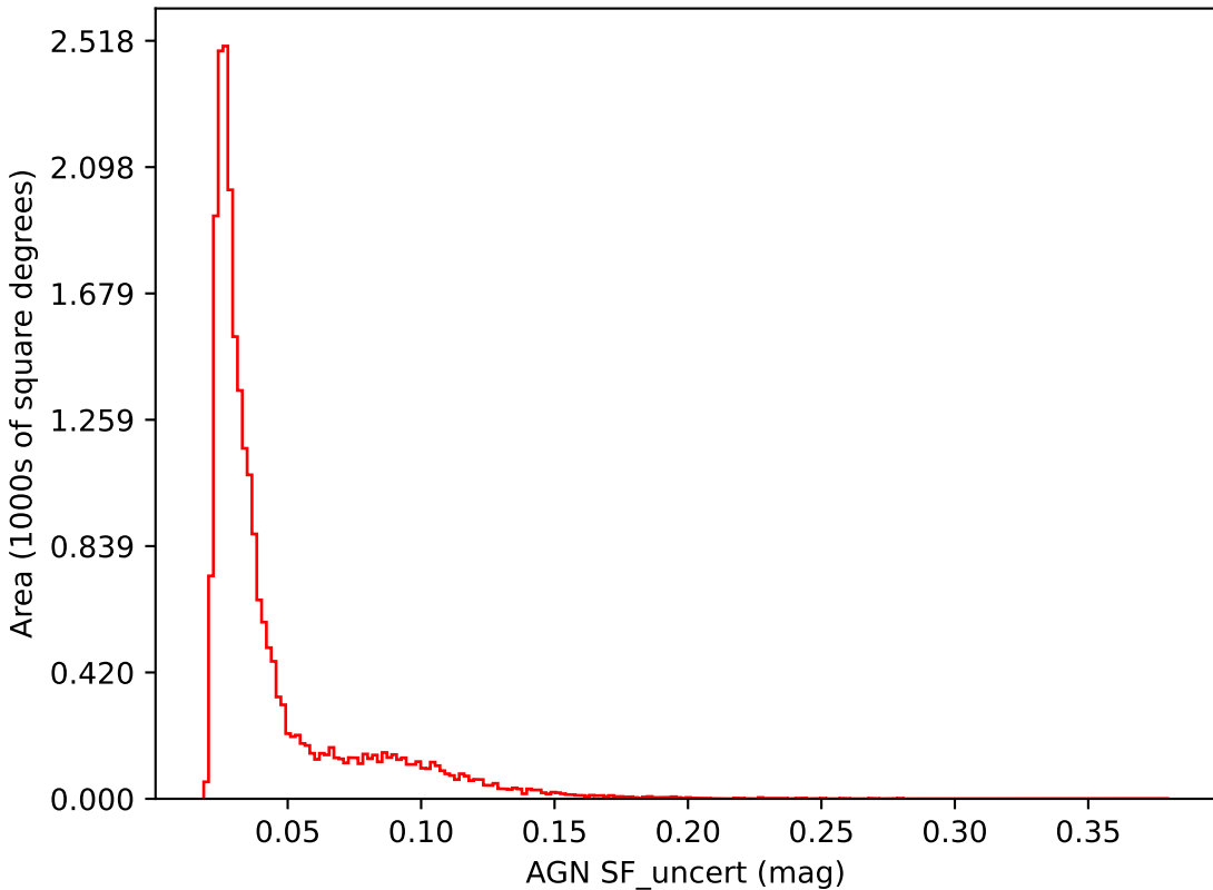
weather_cloudso8v3.4_10yrs i band: AGN SF_uncert
