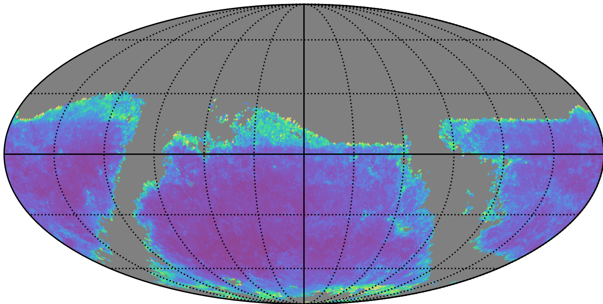
weather_cloudso8v3.4_10yrs g band: AGN SF_uncert
