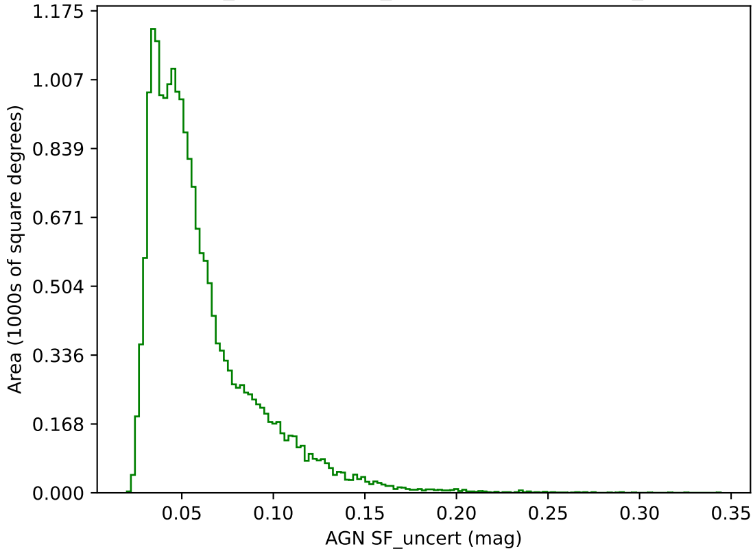
weather_cloudso8v3.4_10yrs g band: AGN SF_uncert
