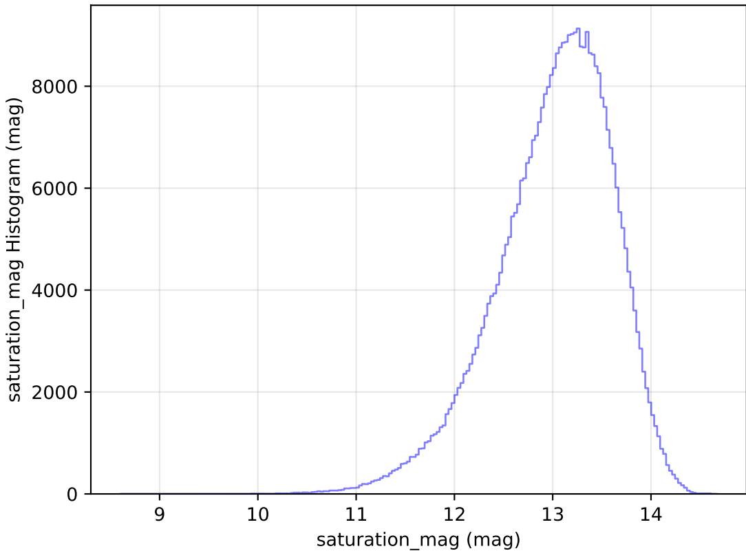
weather_cloudso8v3.4_10yrs WFD y band: saturation_mag Histogram
