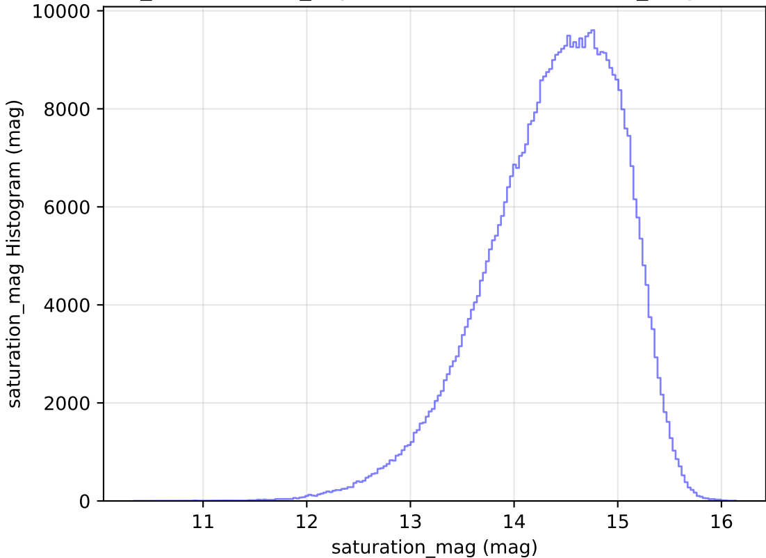
weather_cloudso8v3.4_10yrs WFD i band: saturation_mag Histogram
