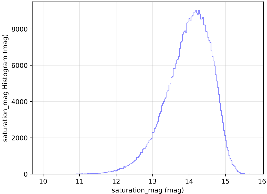
weather_cloudso8v3.4_10yrs All sky z band: saturation_mag Histogram
