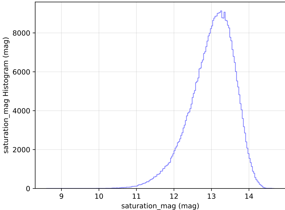
weather_cloudso8v3.4_10yrs All sky y band: saturation_mag Histogram
