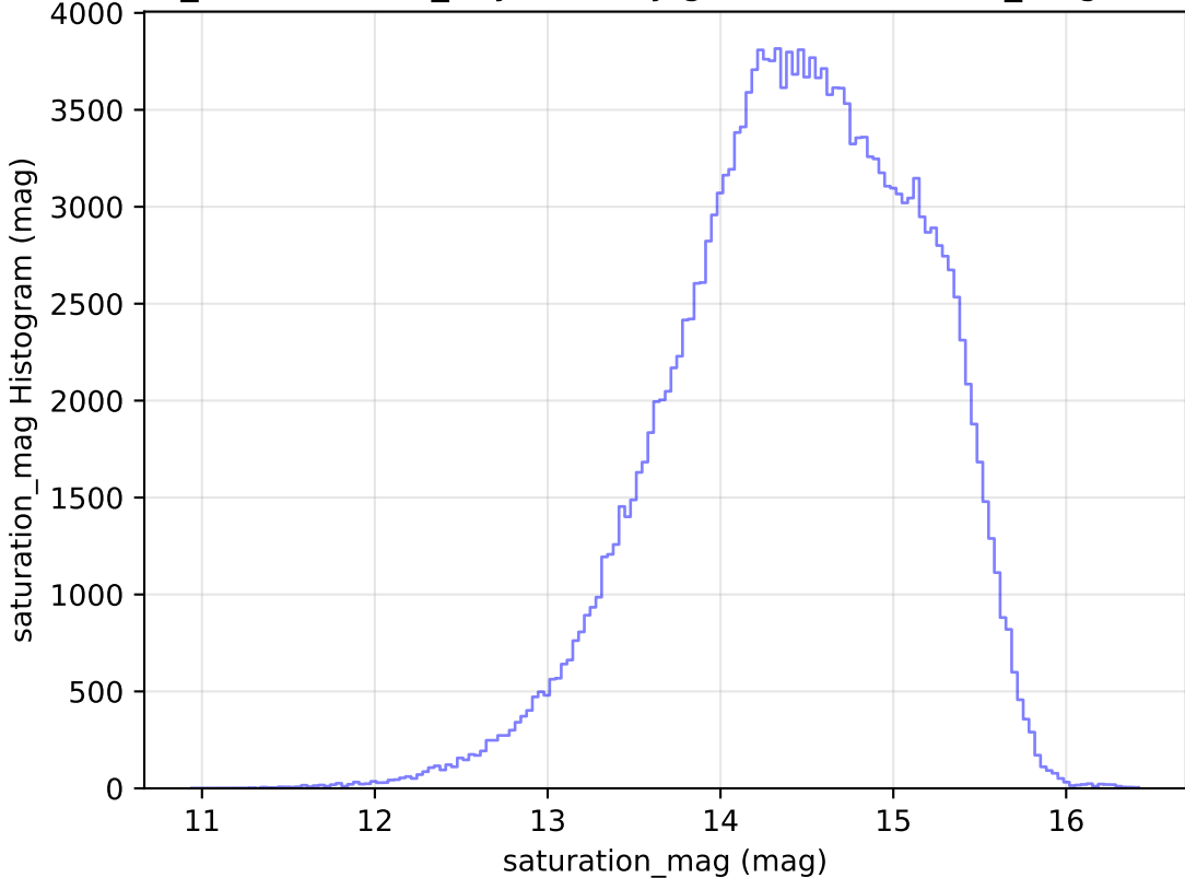
weather_cloudso8v3.4_10yrs All sky g band: saturation_mag Histogram
