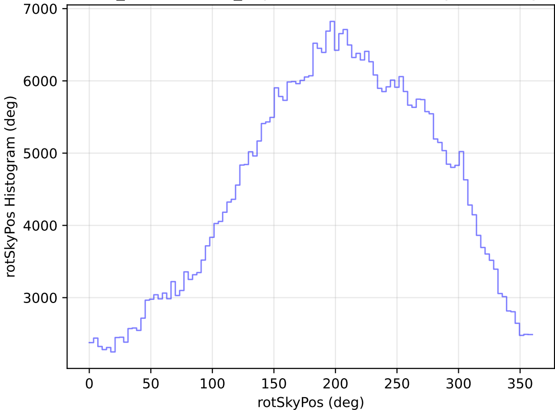
weather_cloudso8v3.4_10yrs WFD z band: rotSkyPos Histogram
