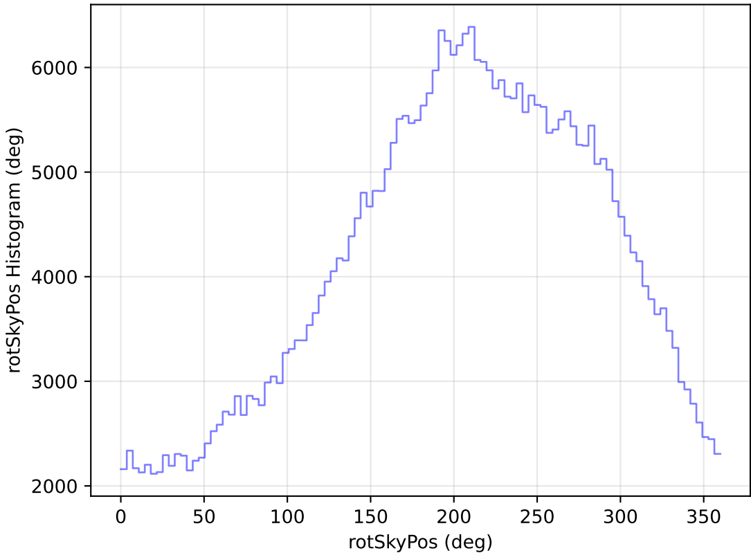
weather_cloudso8v3.4_10yrs WFD y band: rotSkyPos Histogram
