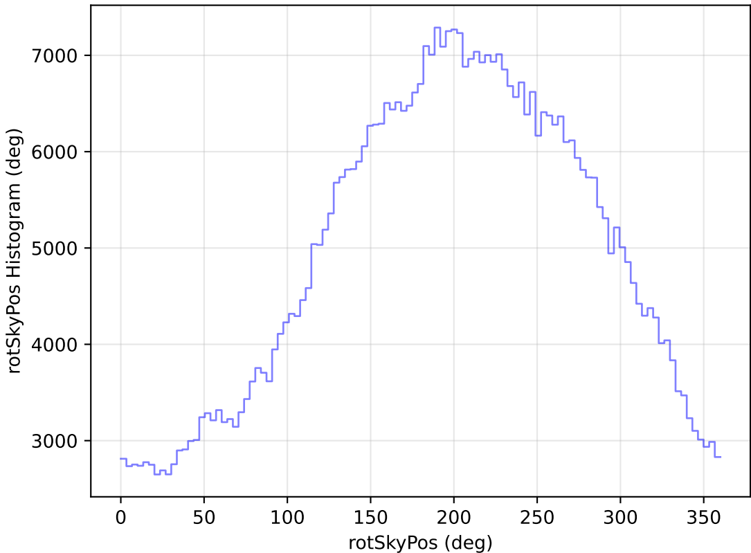
weather_cloudso8v3.4_10yrs WFD i band: rotSkyPos Histogram
