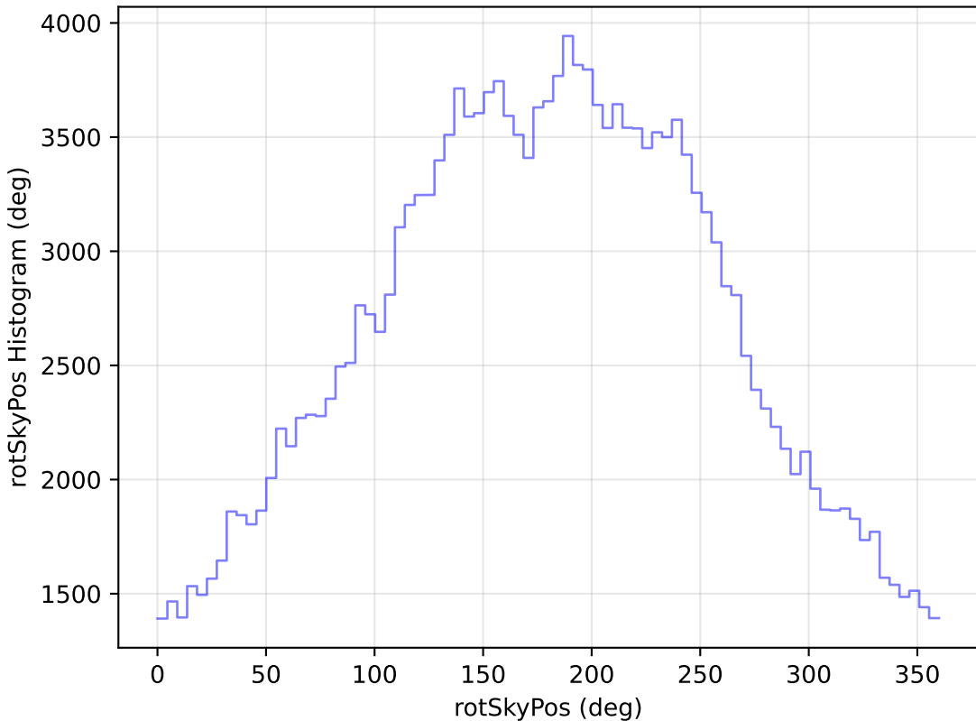
weather_cloudso8v3.4_10yrs WFD g band: rotSkyPos Histogram
