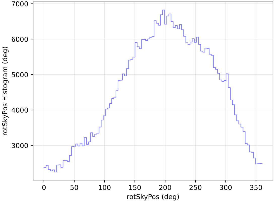
weather_cloudso8v3.4_10yrs All sky z band: rotSkyPos Histogram
