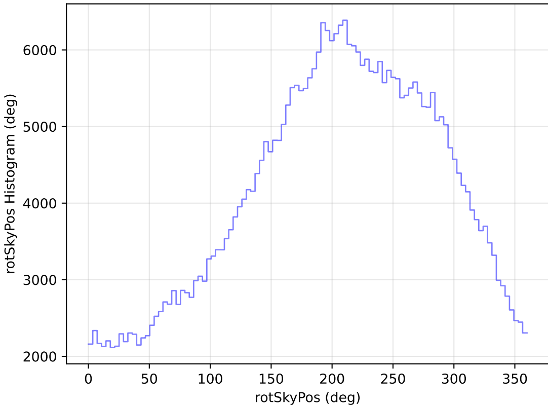
weather_cloudso8v3.4_10yrs All sky y band: rotSkyPos Histogram
