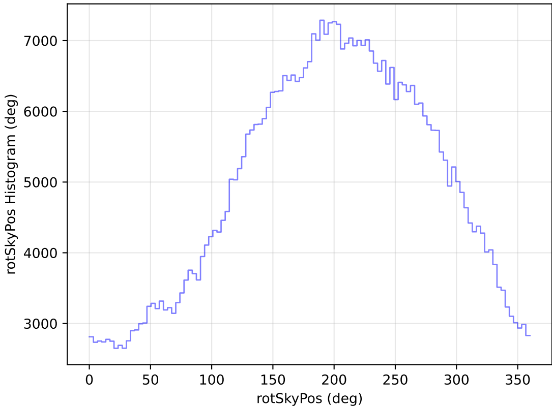
weather_cloudso8v3.4_10yrs All sky i band: rotSkyPos Histogram
