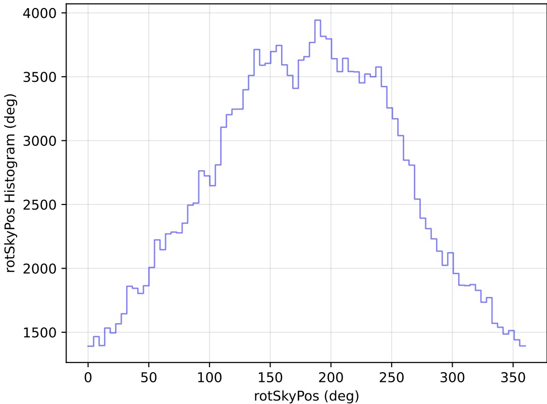
weather_cloudso8v3.4_10yrs All sky g band: rotSkyPos Histogram
