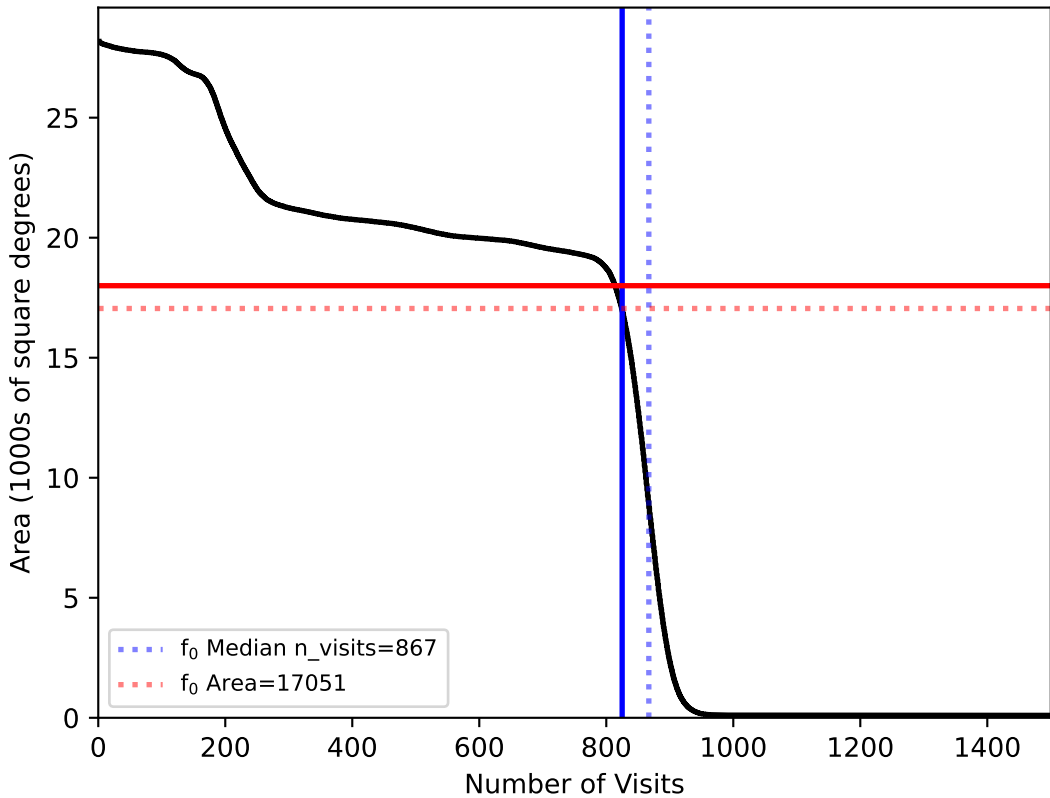
weather_cloudso8v3.4_10yrs All sky: f0
