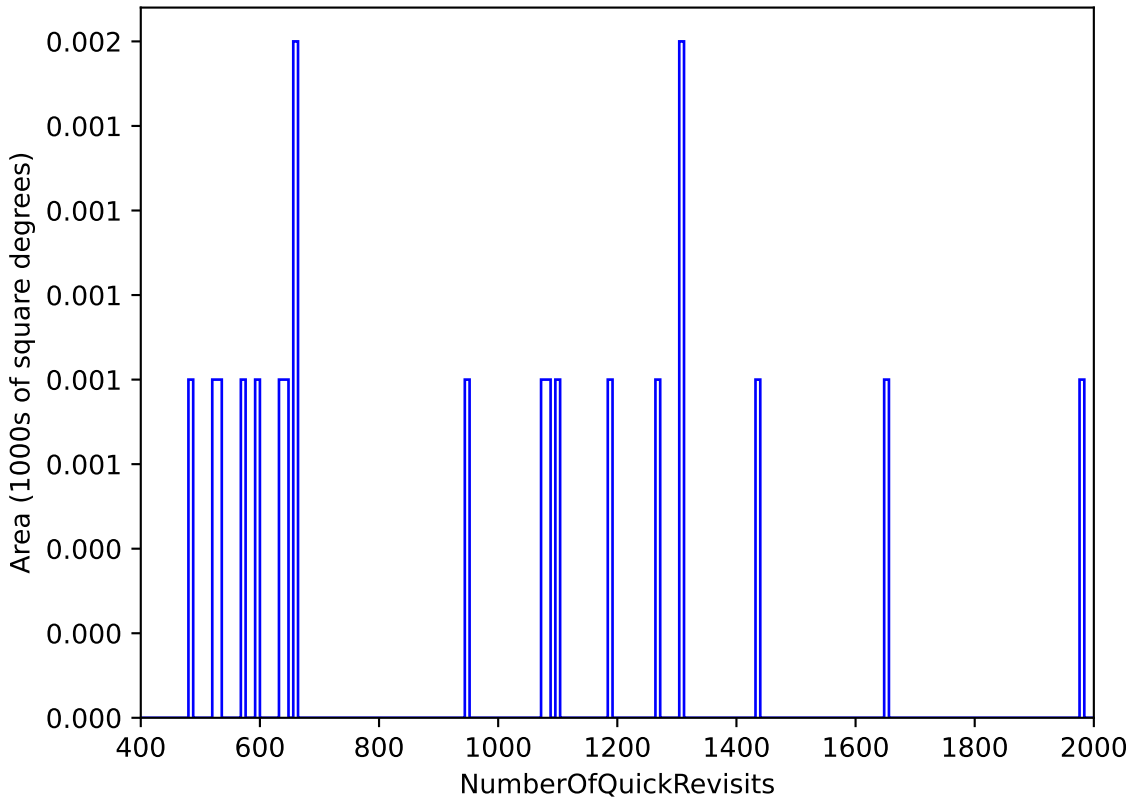
weather_cloudso8v3.4_10yrs All sky: NumberOfQuickRevisits
