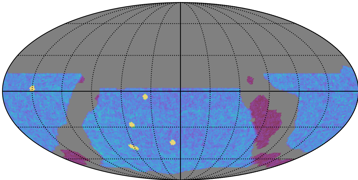
weather_cloudso8v3.4_10yrs WFD y band: NVisits
