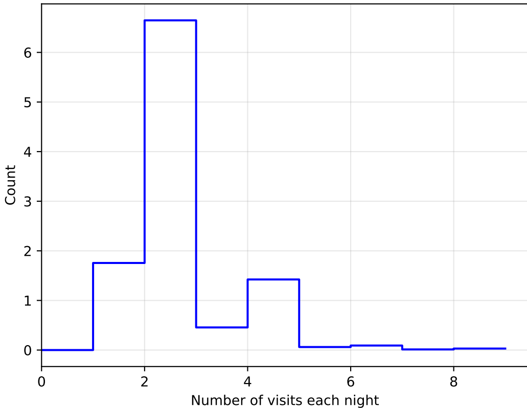
1e6 weather_cloudso8v3.4_10yrs All sky: NVisitsPerNight
