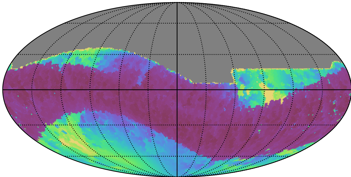
weather_cloudso8v3.4_10yrs All sky i band: Min solarElong
