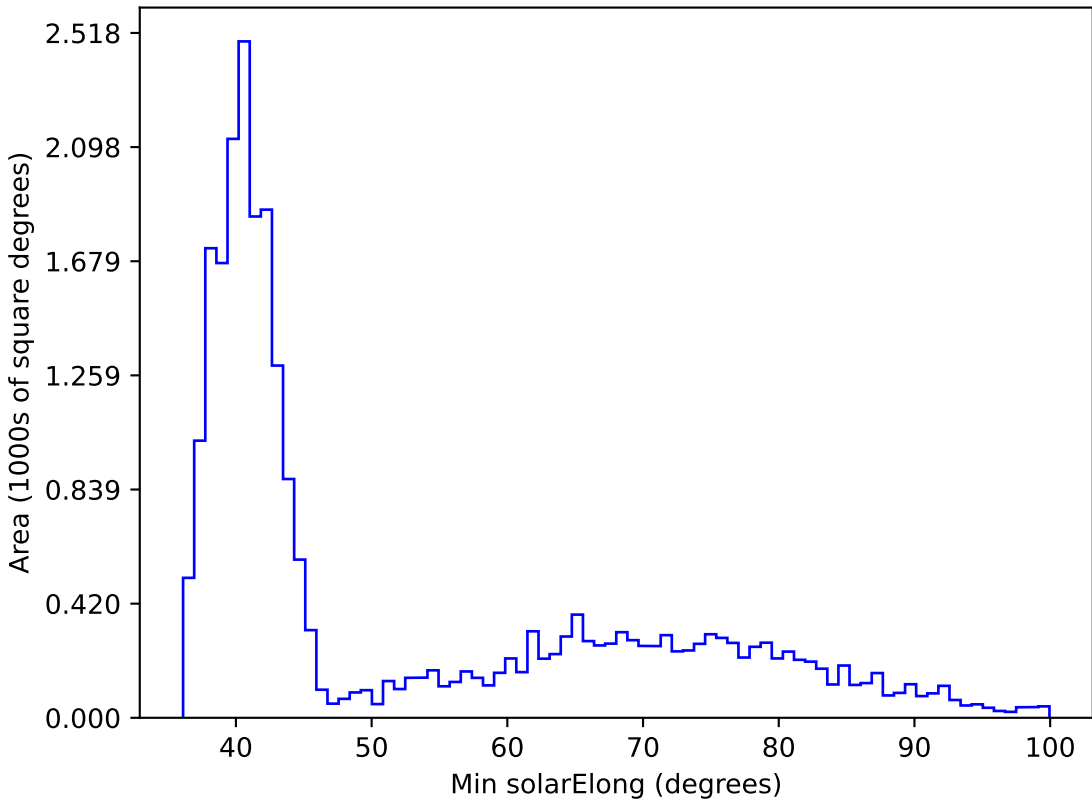
weather_cloudso8v3.4_10yrs All sky i band: Min solarElong
