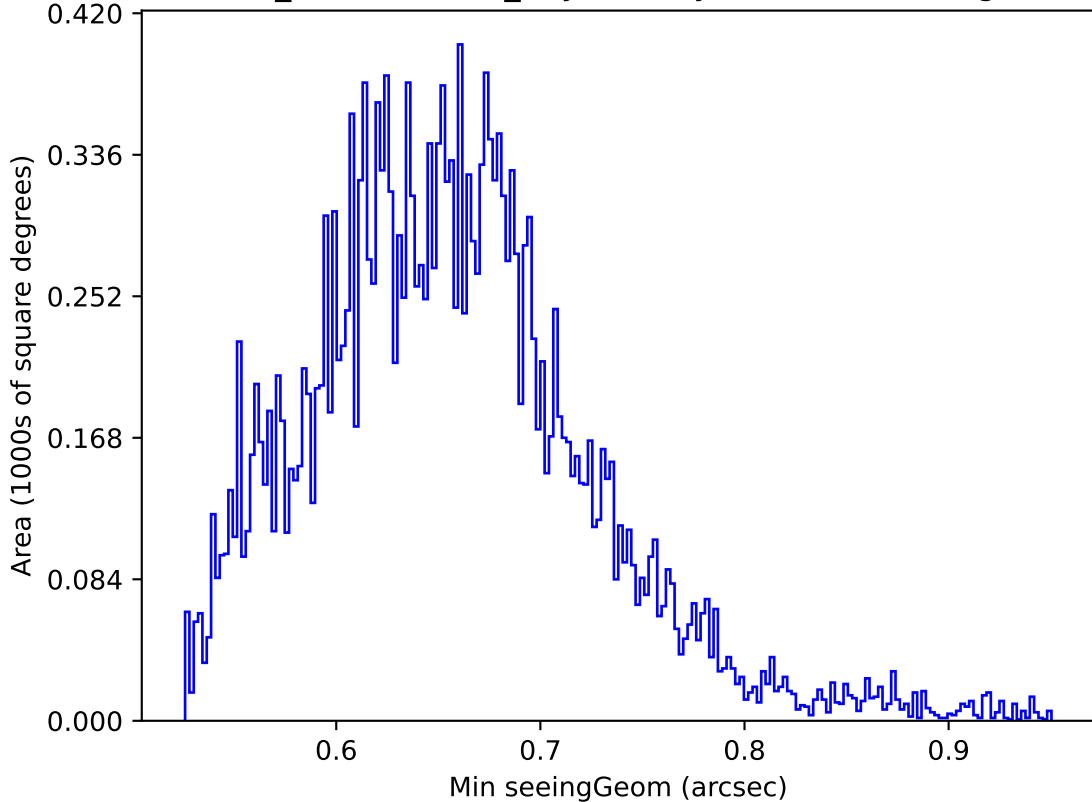
weather_cloudso8v3.4_10yrs Yr 1 y band: Min seeingGeom
