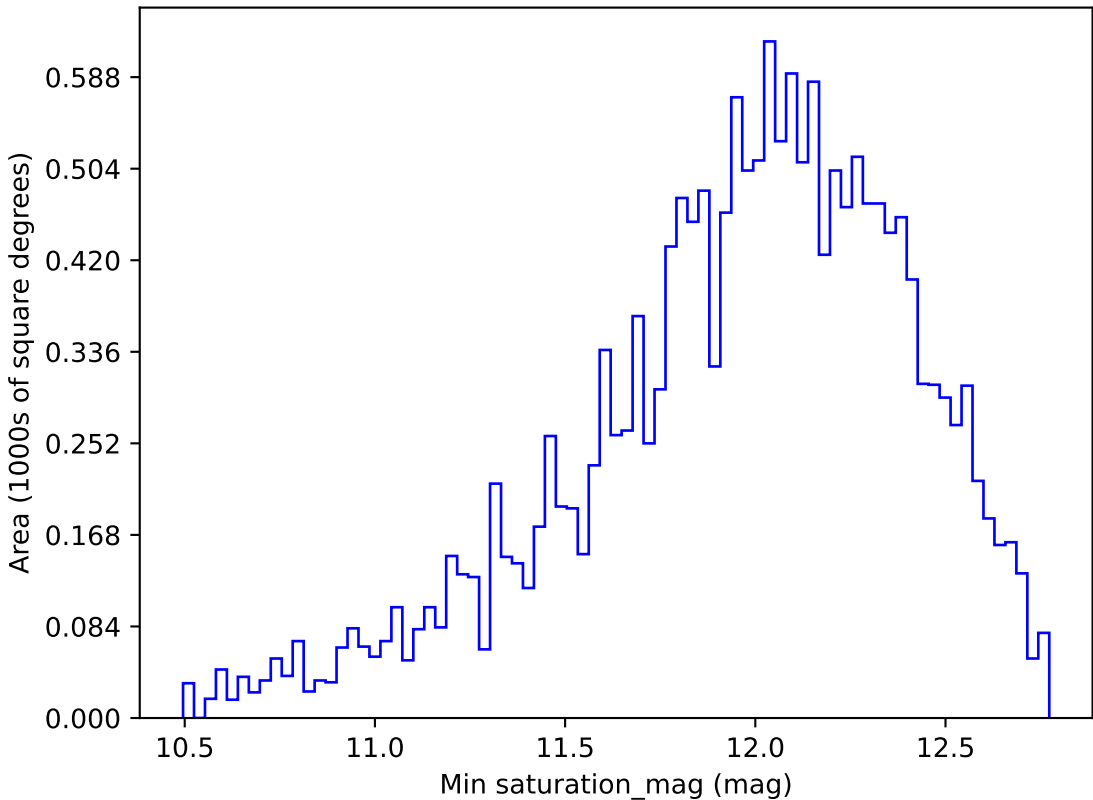
weather_cloudso8v3.4_10yrs WFD z band: Min saturation_mag
