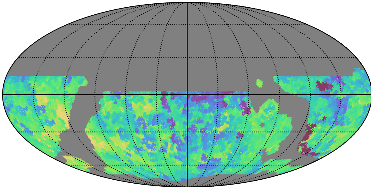
weather_cloudso8v3.4_10yrs WFD y band: Min saturation_mag
