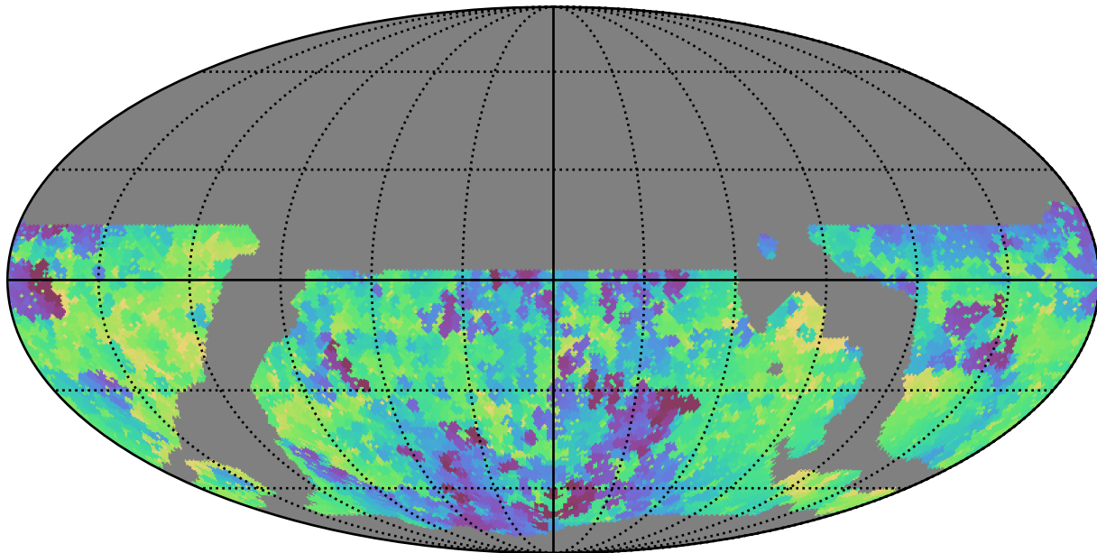
weather_cloudso8v3.4_10yrs WFD u band: Min saturation_mag
