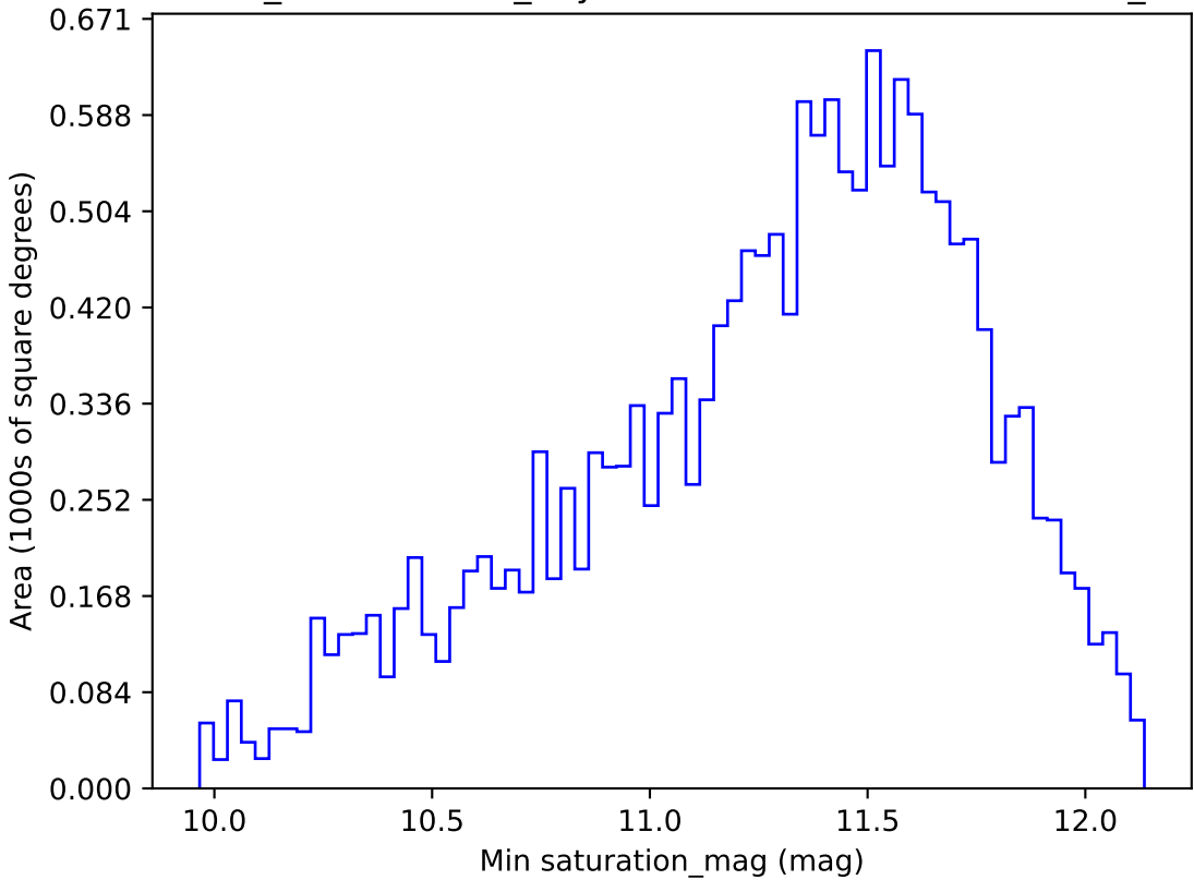
weather_cloudso8v3.4_10yrs WFD u band: Min saturation_mag
