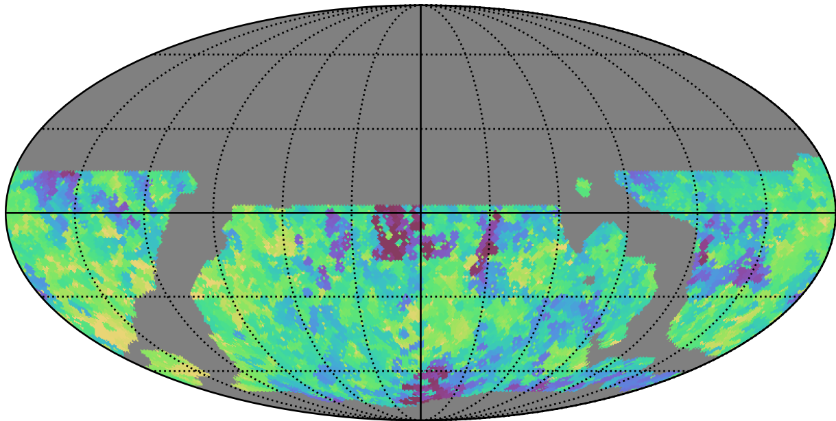
weather_cloudso8v3.4_10yrs WFD i band: Min saturation_mag
