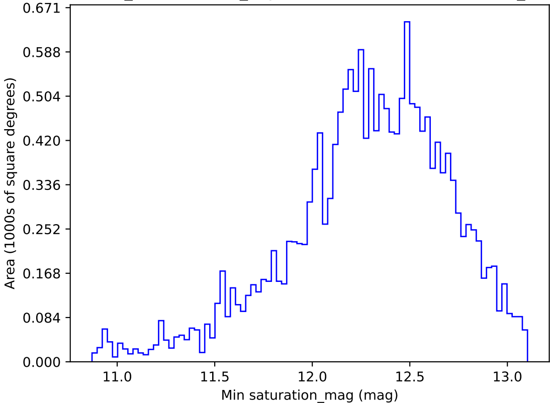
weather_cloudso8v3.4_10yrs WFD i band: Min saturation_mag
