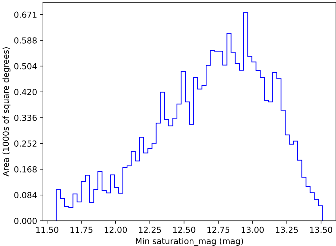
weather_cloudso8v3.4_10yrs WFD g band: Min saturation_mag
