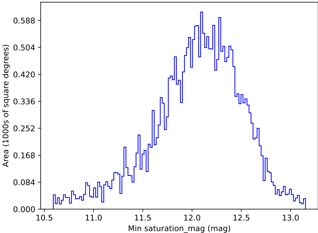
weather_cloudso8v3.4_10yrs All sky z band: Min saturation_mag
