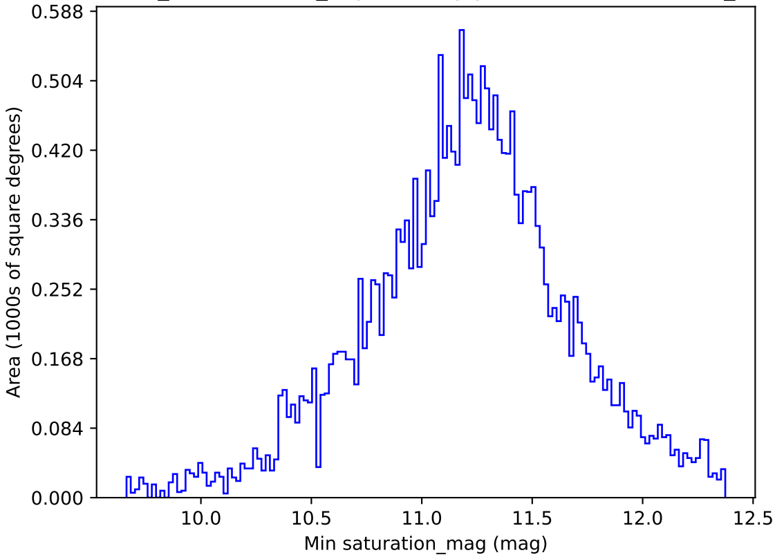
weather_cloudso8v3.4_10yrs All sky y band: Min saturation_mag
