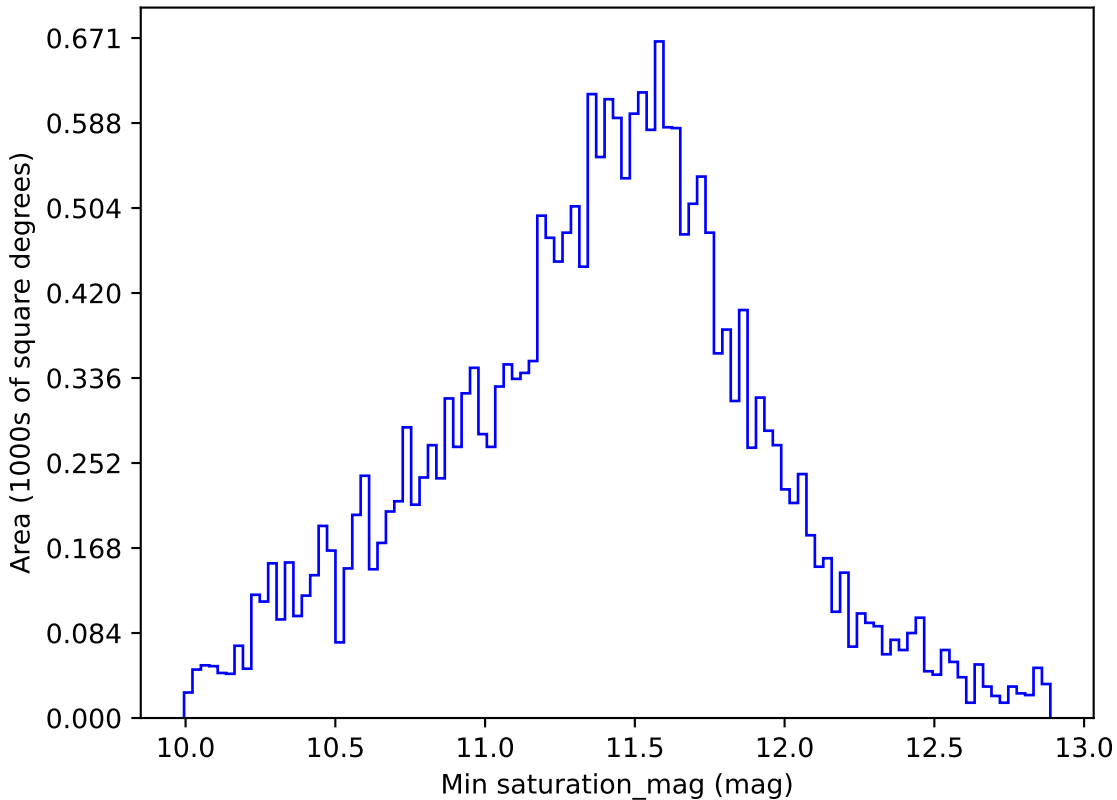
weather_cloudso8v3.4_10yrs All sky u band: Min saturation_mag
